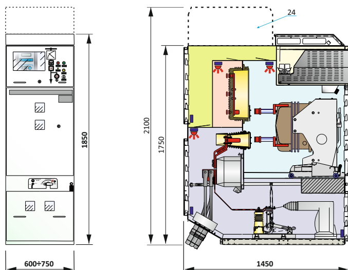
Pole rozdzielnic z przedziałem obwodów pomocniczych w wersji wysuwnej Panel of switchgear with auxiliary circuits compartment in withdrawable version
