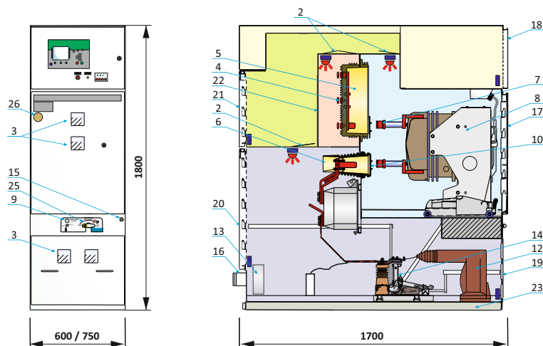
Pole rozdzielcze rozdzielnic PREM-G1dM w wersji 1800 mm wysokości Distribution panel of the PREM-G1dM switchgear in the 1800 mm height version
