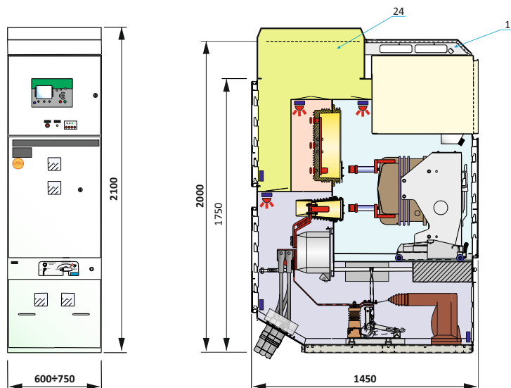
Pole rozdzielnic z przedziałem obwodów pomocniczych w wersji stacjonarnej Panel of switchgear with auxiliary circuits compartment in stationary version
