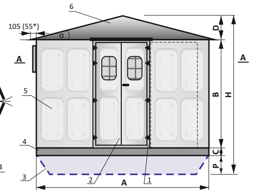
Widok ściany czołowej stacji SKP Front wall view of the SKP substation
