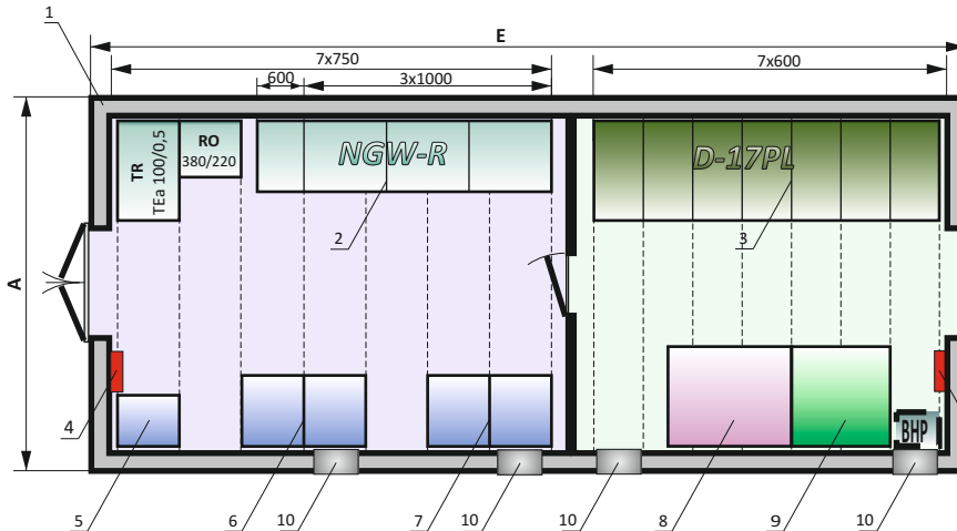
Przykład rozmieszczenia urządzeń w stacji SKP (przekrój A-A) Example of equipment lay-out in the SKP substation (section view A-A)
